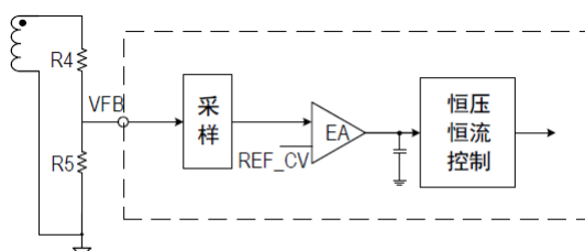
图4：恒压工作原理图
